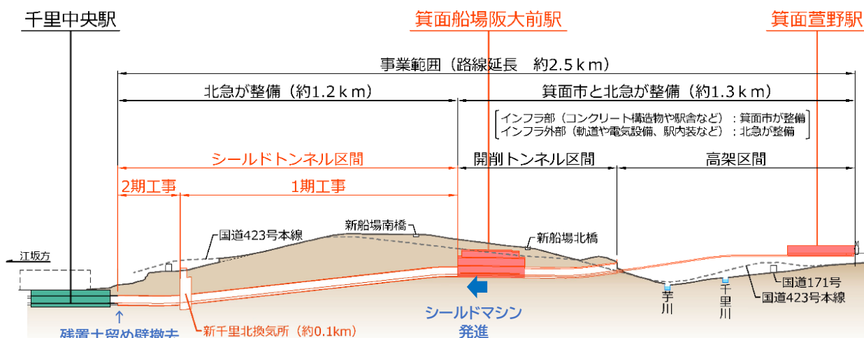
北大阪急行線の延伸工事のうち土木工事 縦断面図 (千里中央駅～箕面船場阪大前駅間の残置土留め壁撤去、シールドトンネル工事)
